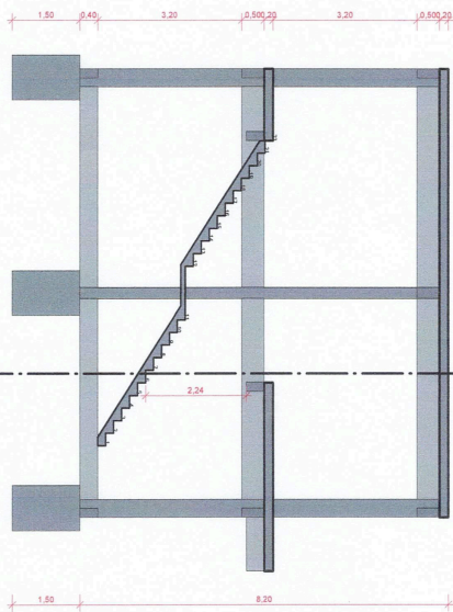
B Corte B-B ESCALA 1/75
