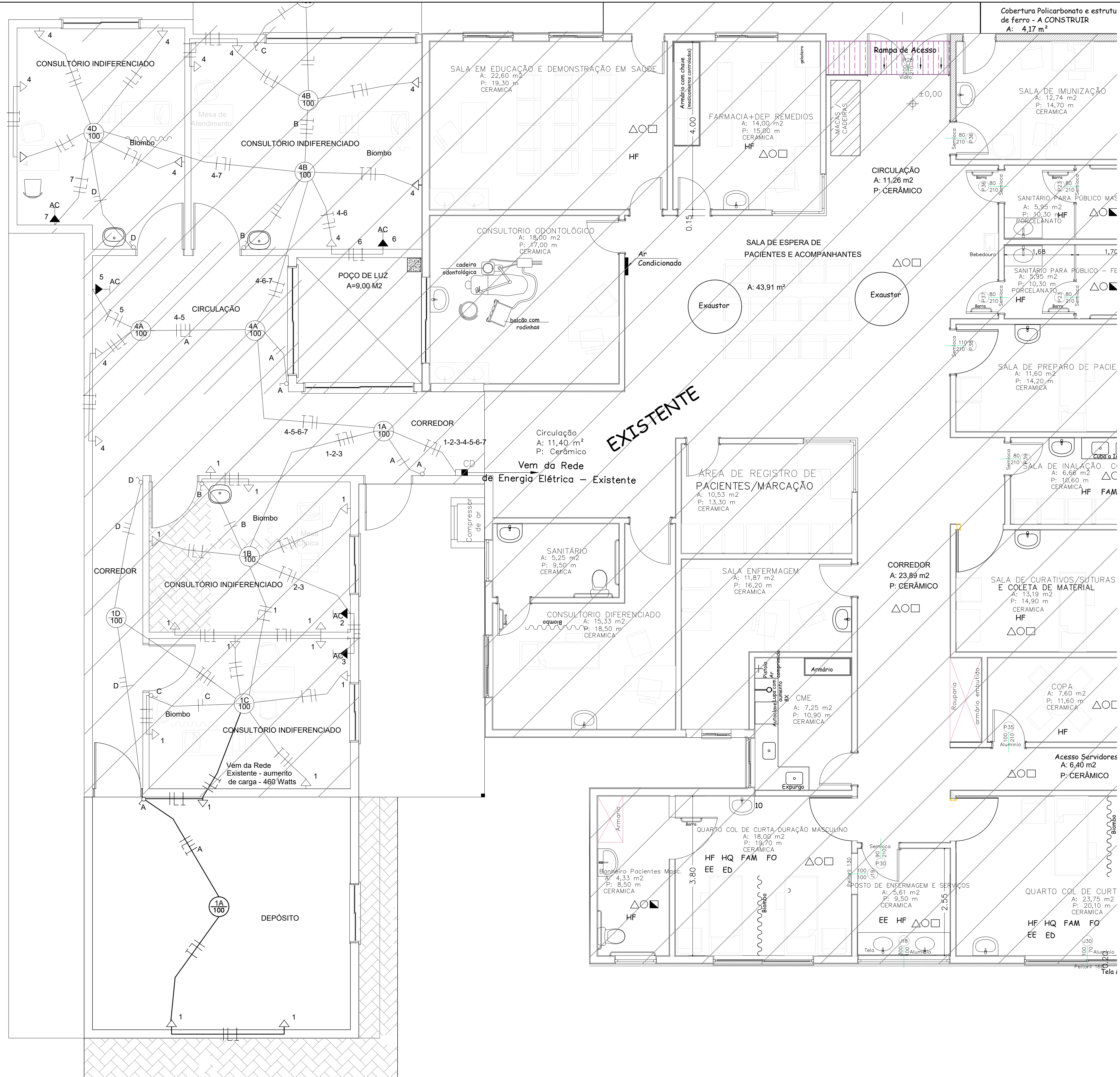
08 PLANTA ELÉTRICA ESCALA: 1/50
